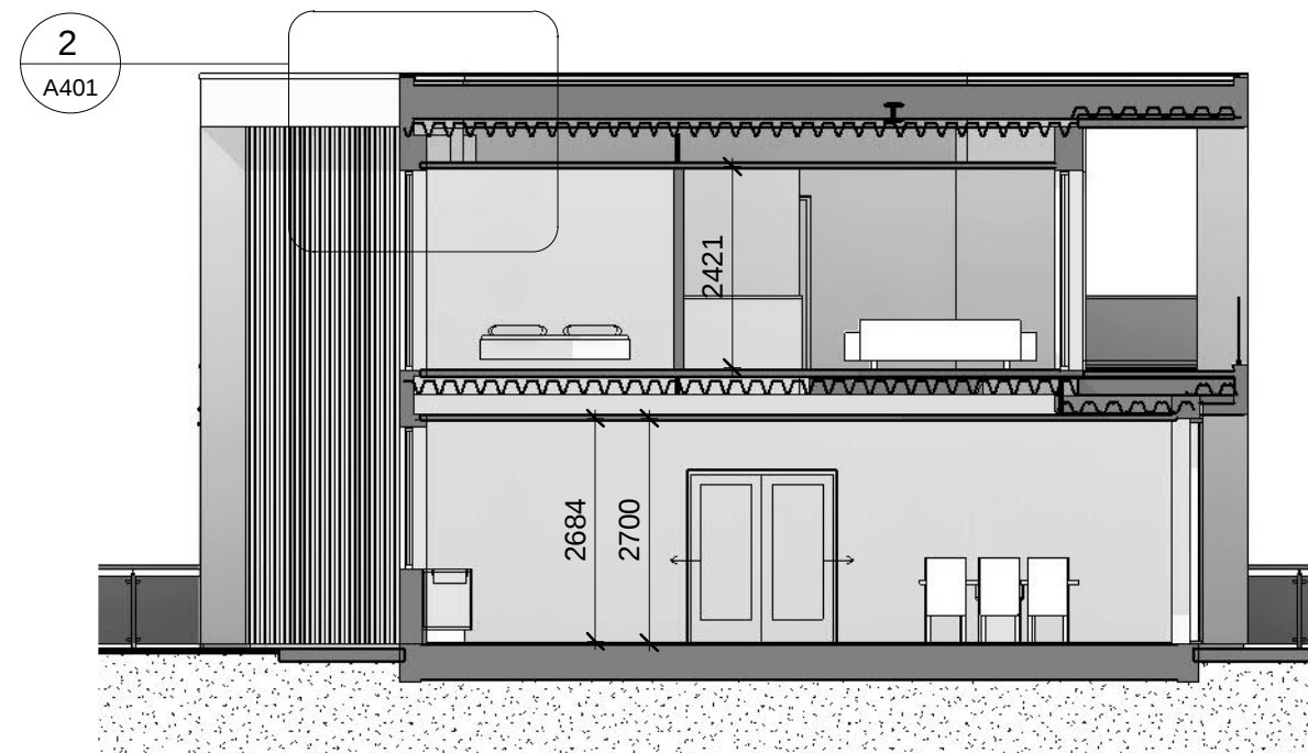
Snitt 3 1 : 100
