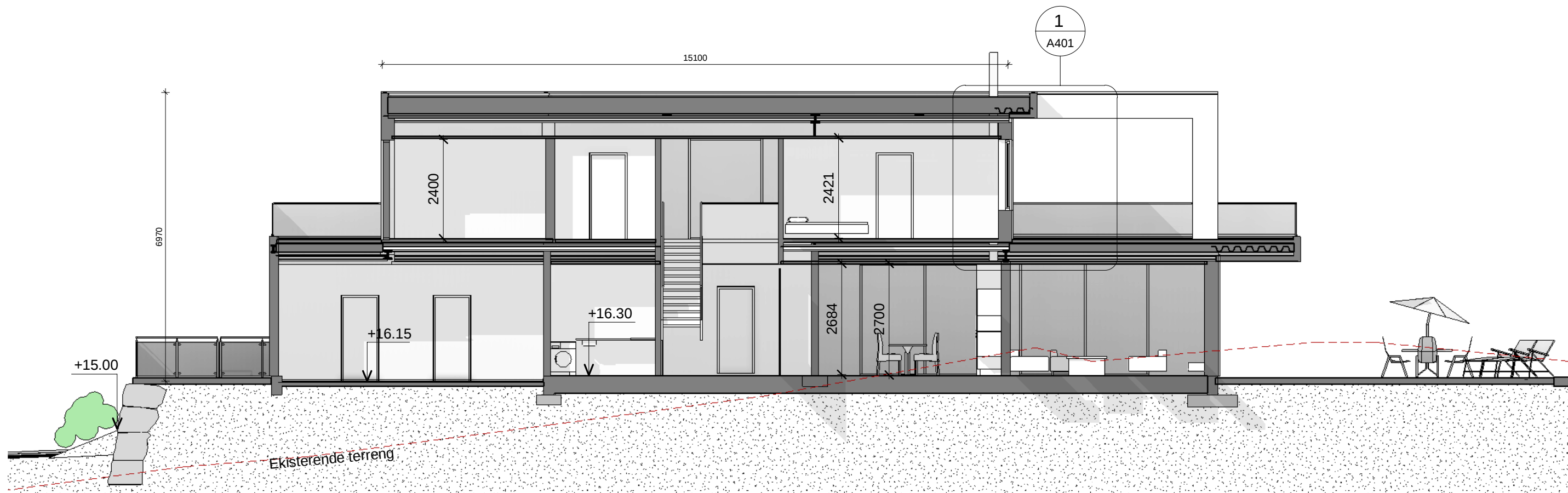
Snitt 1 1 : 100
