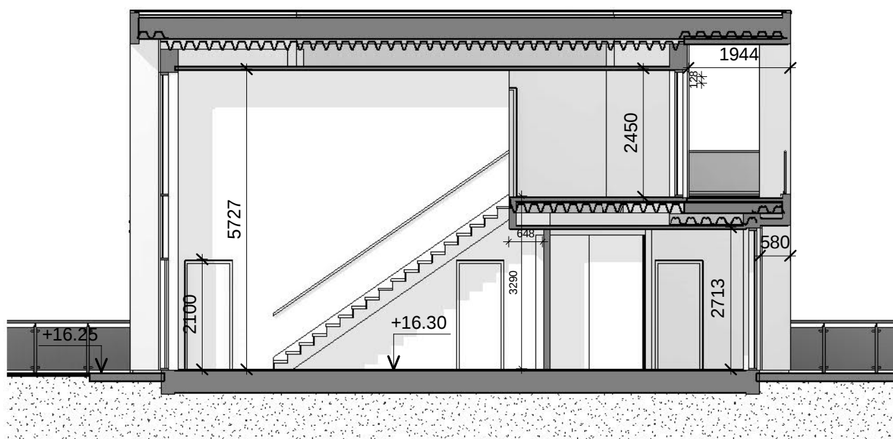
Snitt 2 1 : 100
