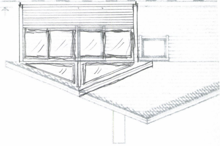
FASADE MOT ÖST
