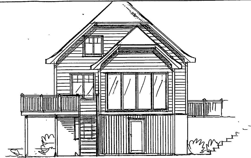
FASADE SØR
