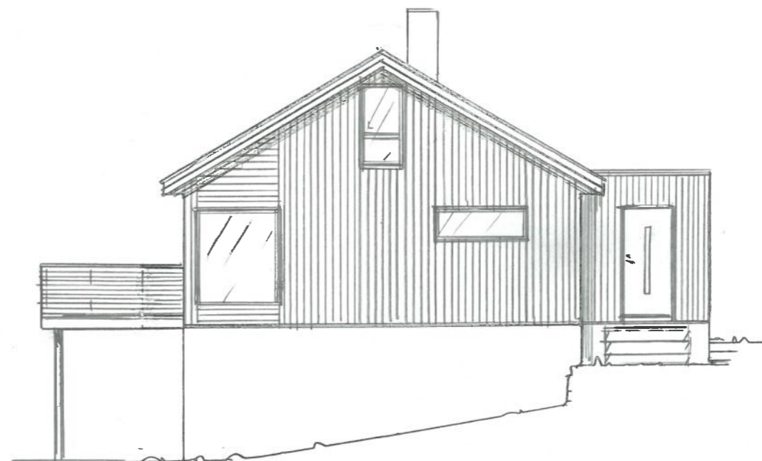
FASADE ØST
