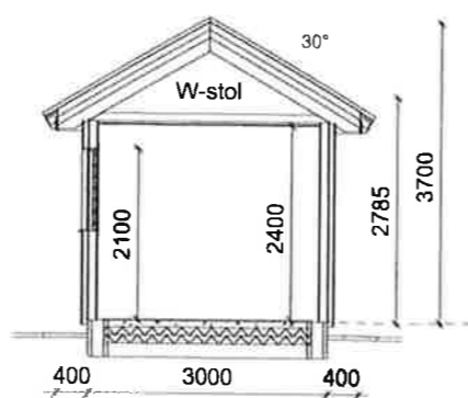
Snitt A-A
