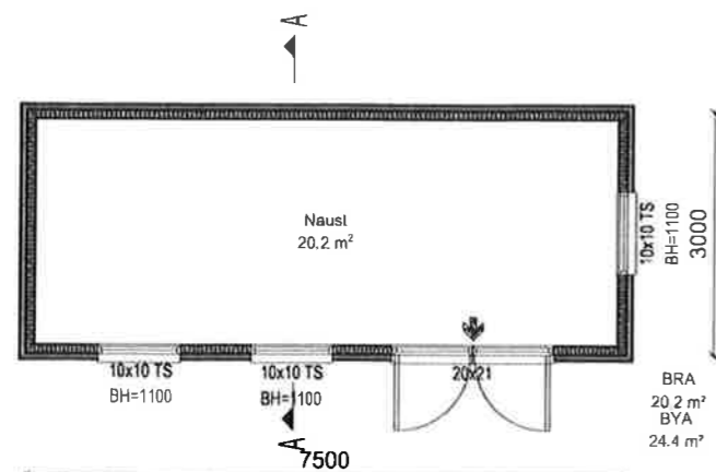
Plan 1 etg.
