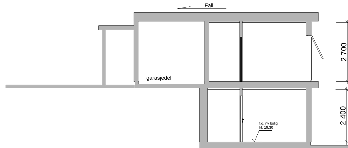
1:100 Snitt A
