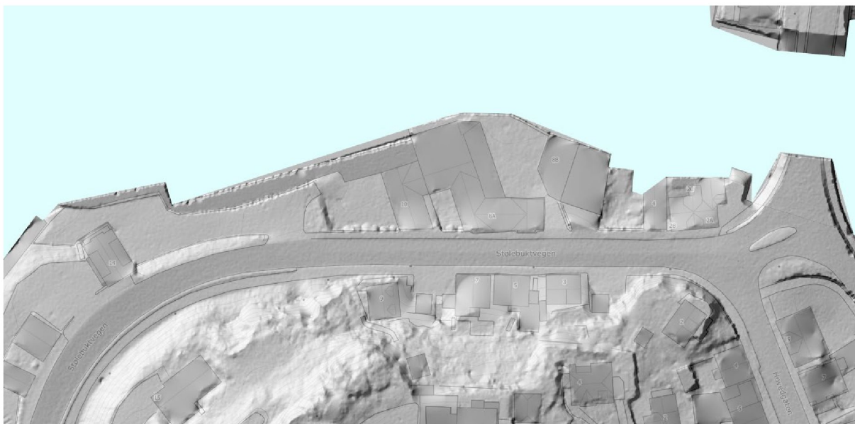
Figur 2: Digital terrengmodell (DTM)
