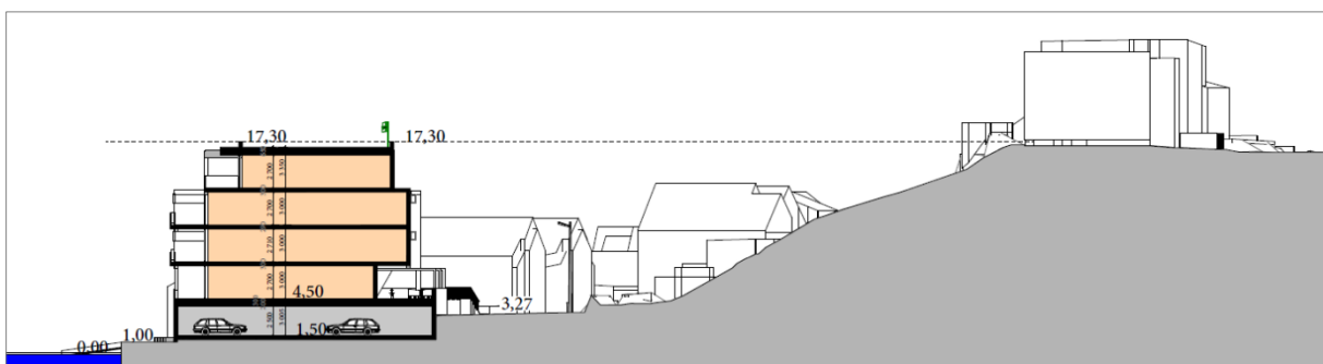
Figur 9: Tverrsnitt av Stølebuktvegen
