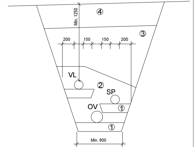
Generellt grøftesnitt
