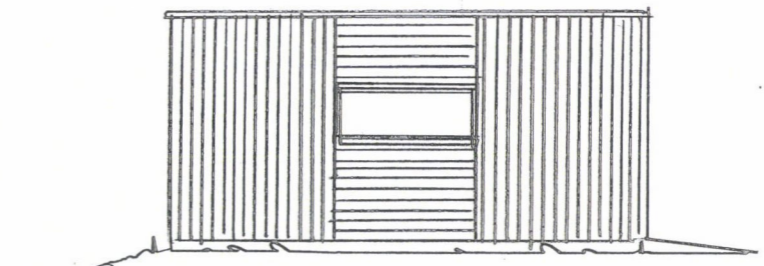
FASADE ØST
