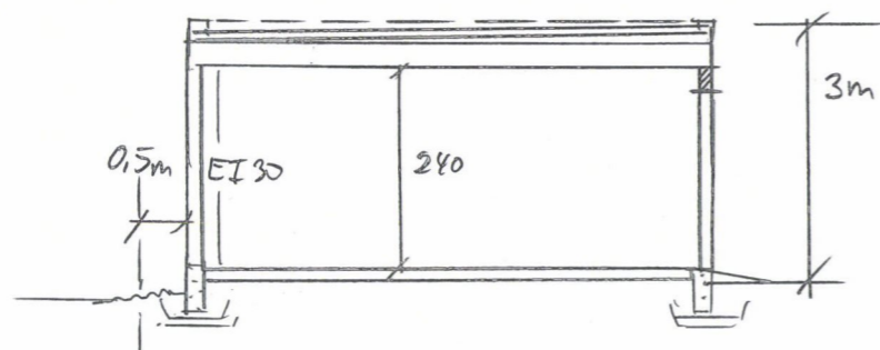
SNITT
