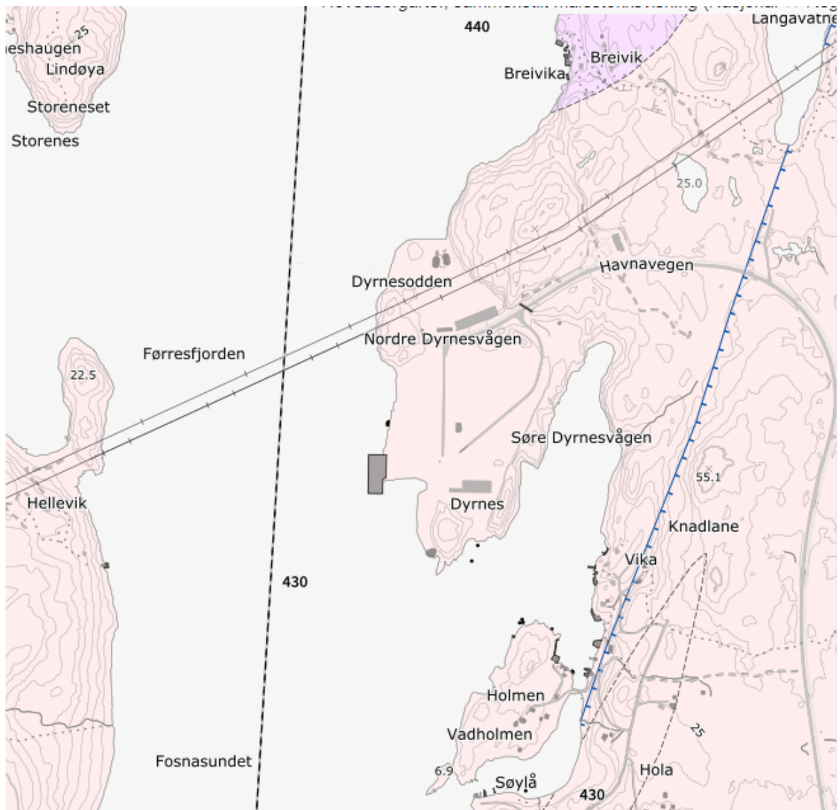
Figur 5-6: Kartet viser berggrunnen på land i tiltaksområdet. Rosa er granittisk øyegneis, middelskornet, øyne av kalifeltspataggregater og Lilla er migmatitt med glimmergneispaleosom. Kilde: NGU
