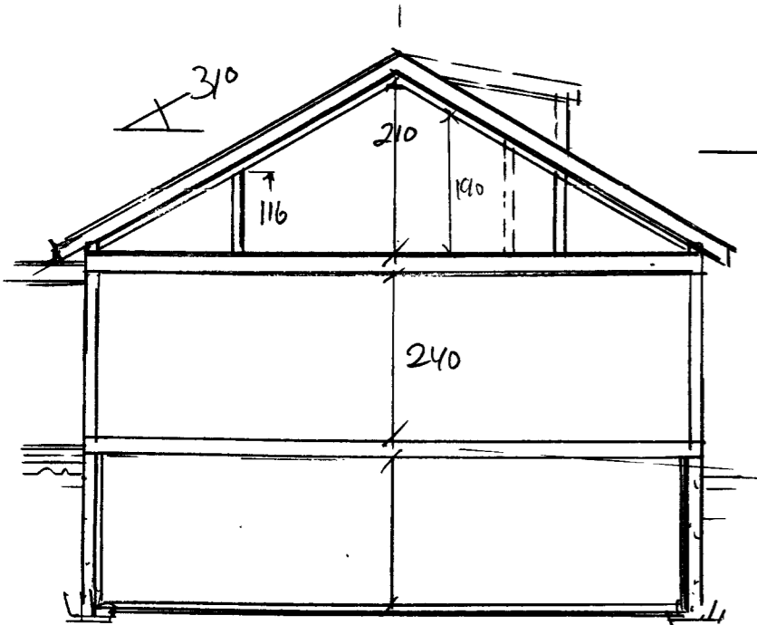
SNITT
