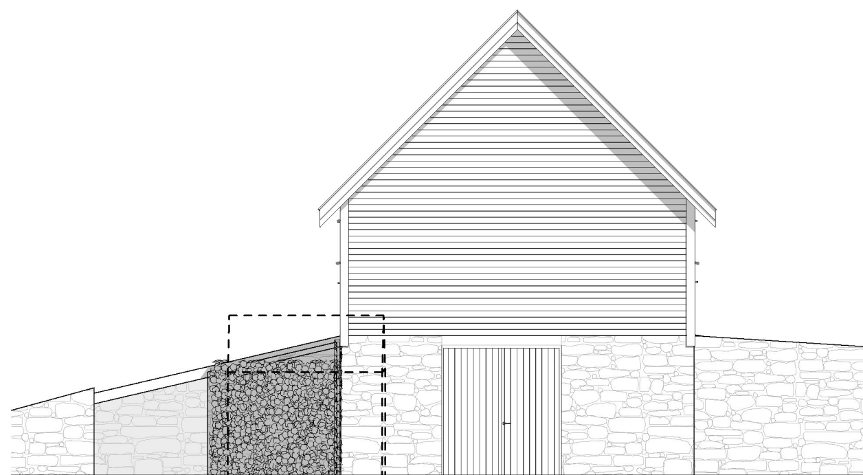
FASADE SØR
