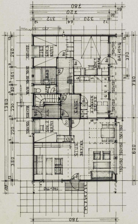
PLAN AV FIASJE
