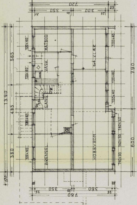
KJELLERPLAN
