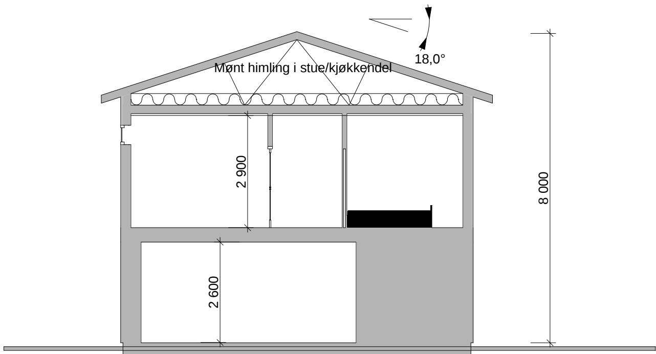
1:100 Snitt A
