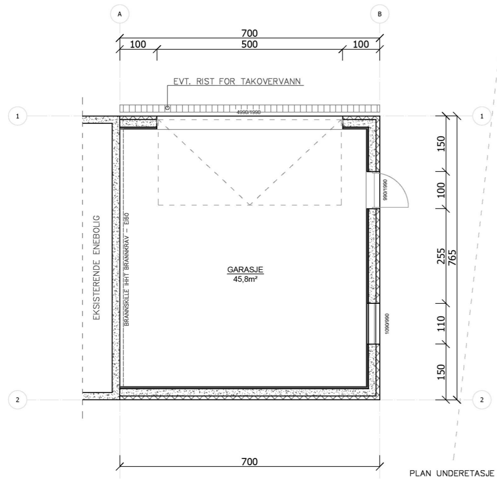
PLAN UNDERETASJE
