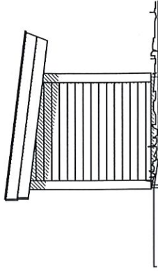
FASADE 3 Nord-Vest
