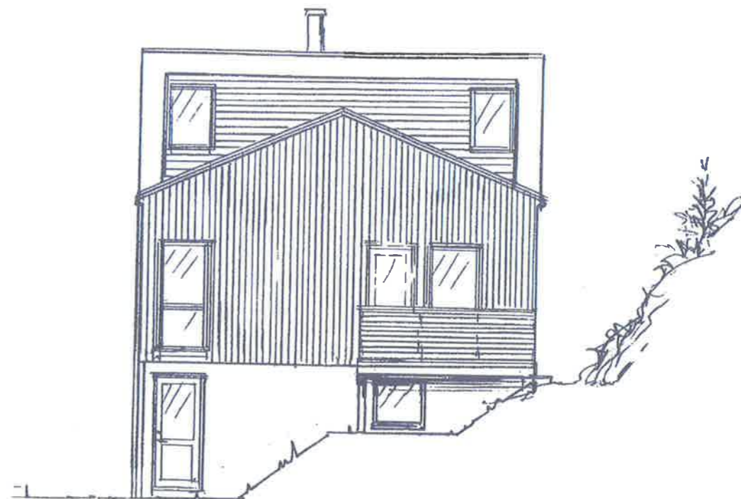
FASADE NORD ØST
