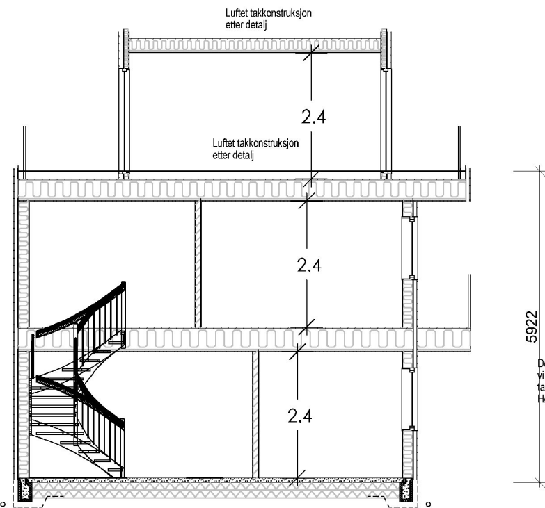
Snitt A:A
