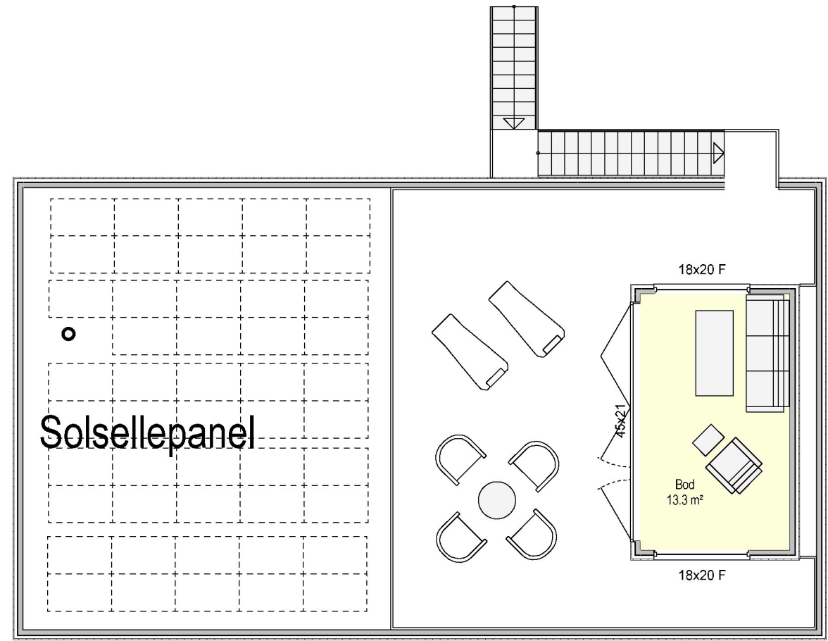
Plan 3 etg
