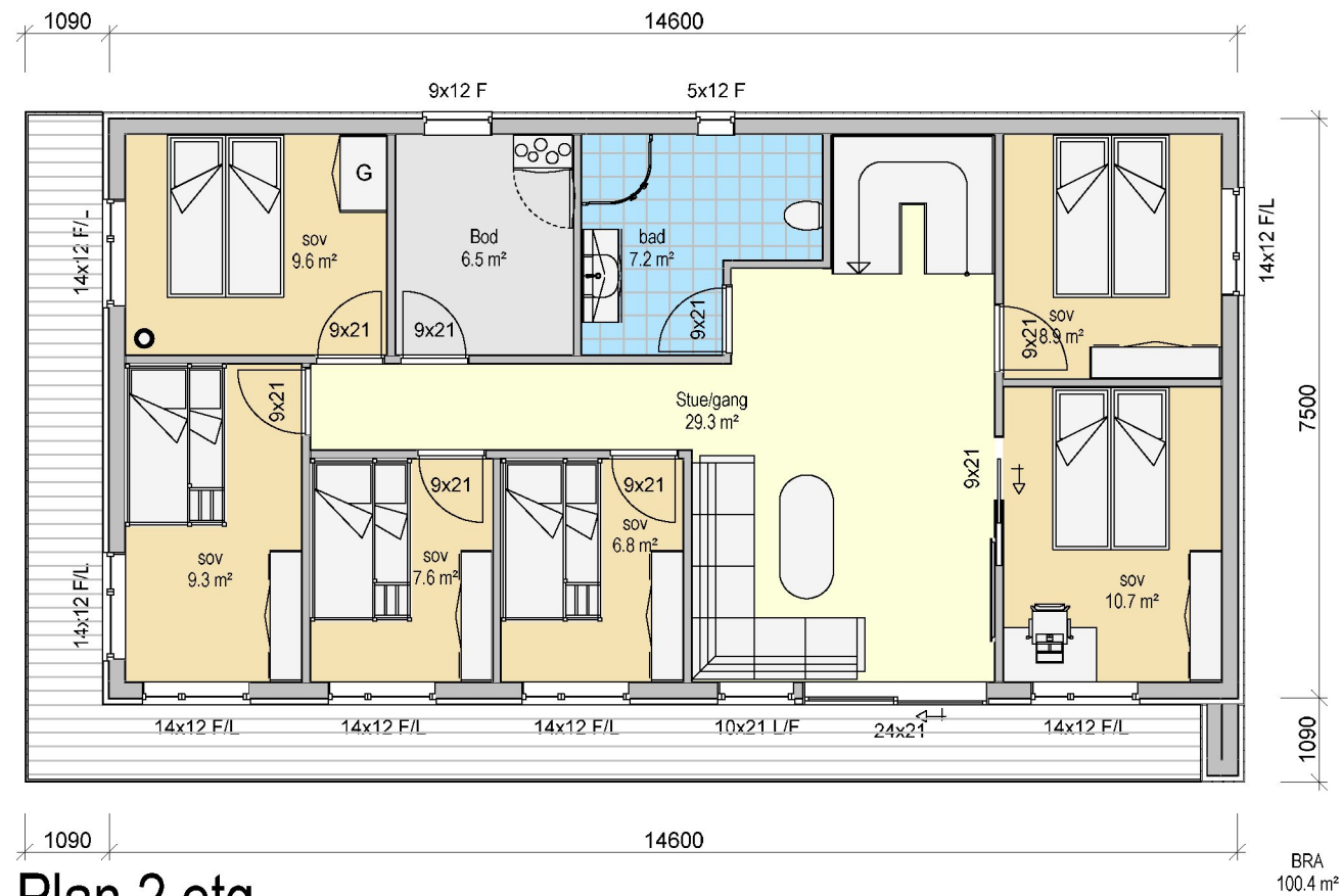
Plan 2 etg
