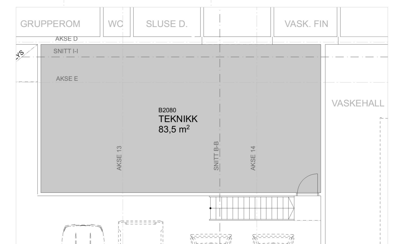
UTSNITT B - PÅ MEZZANIN OVER SLANGEVASK/VERKSTED
