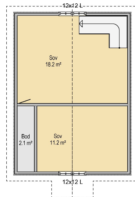
Plan 2 etg
