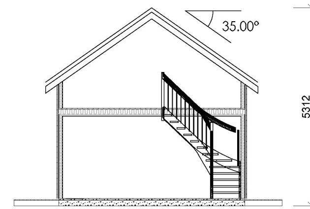
Snitt A:A
