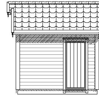
Fasade vest
