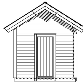
Fasade nord
