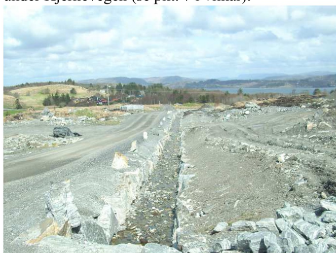
9. Etablert kanalløp langsetter Kjerkevegen (på naboeiendom med gnr./bnr. 118/1).
