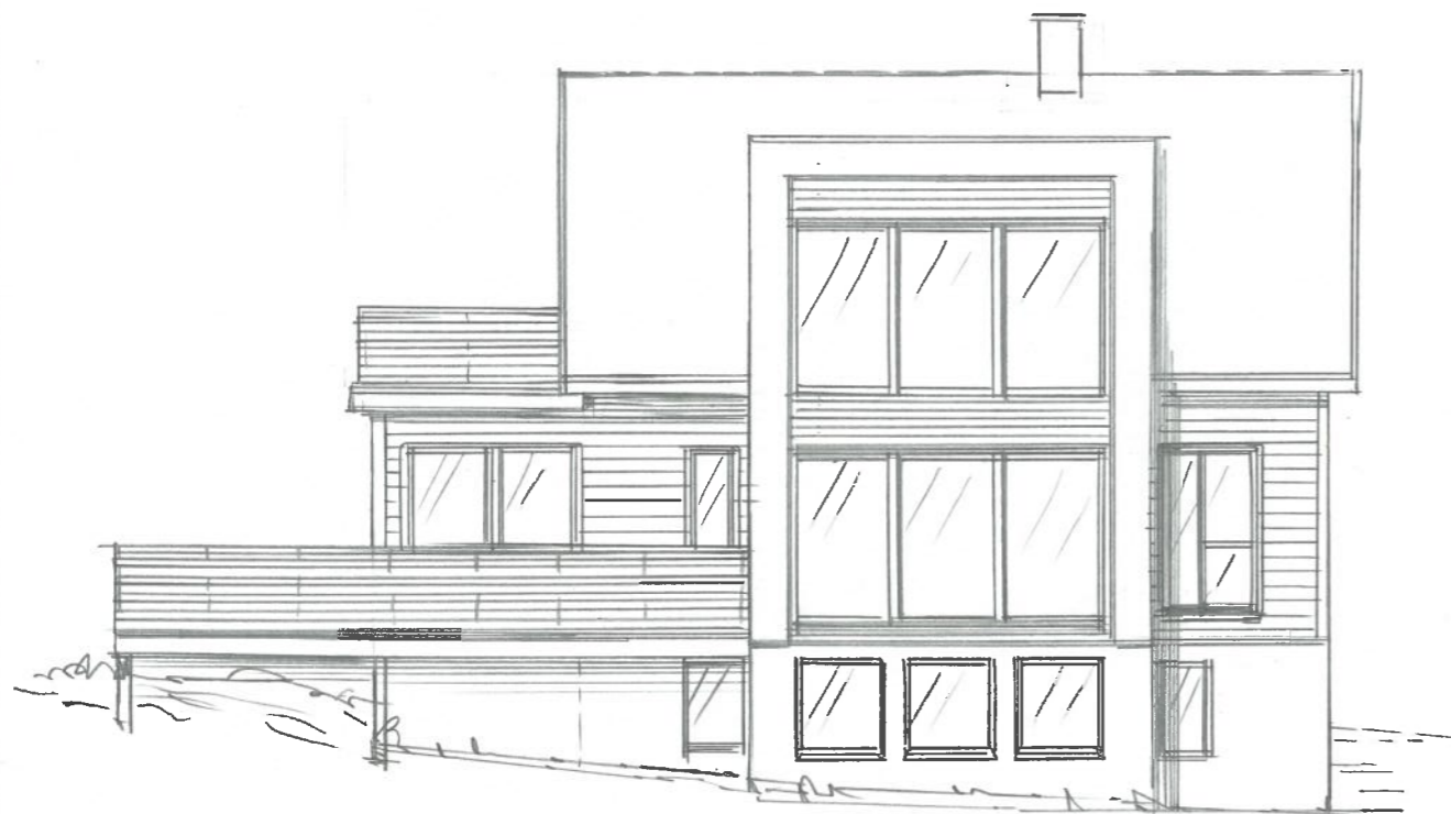
FASADE ØST
