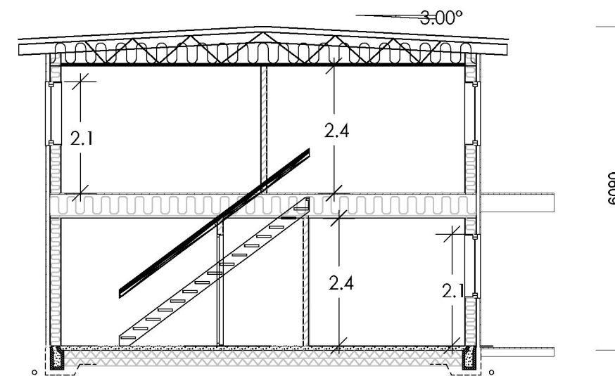
Snitt B:B
