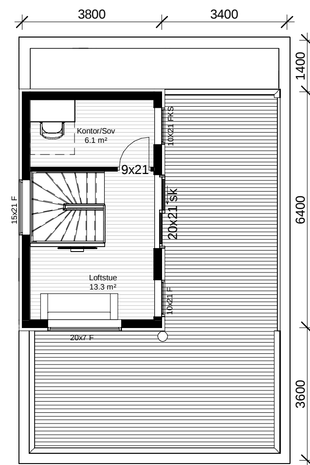
Et. 3 1 : 100
