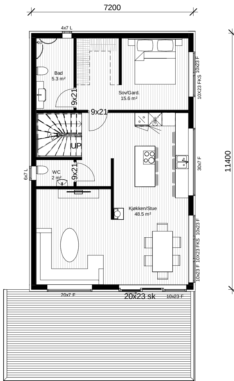
Et. 2 1 : 100
