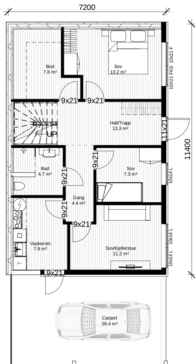
Et. 1 1 : 100
