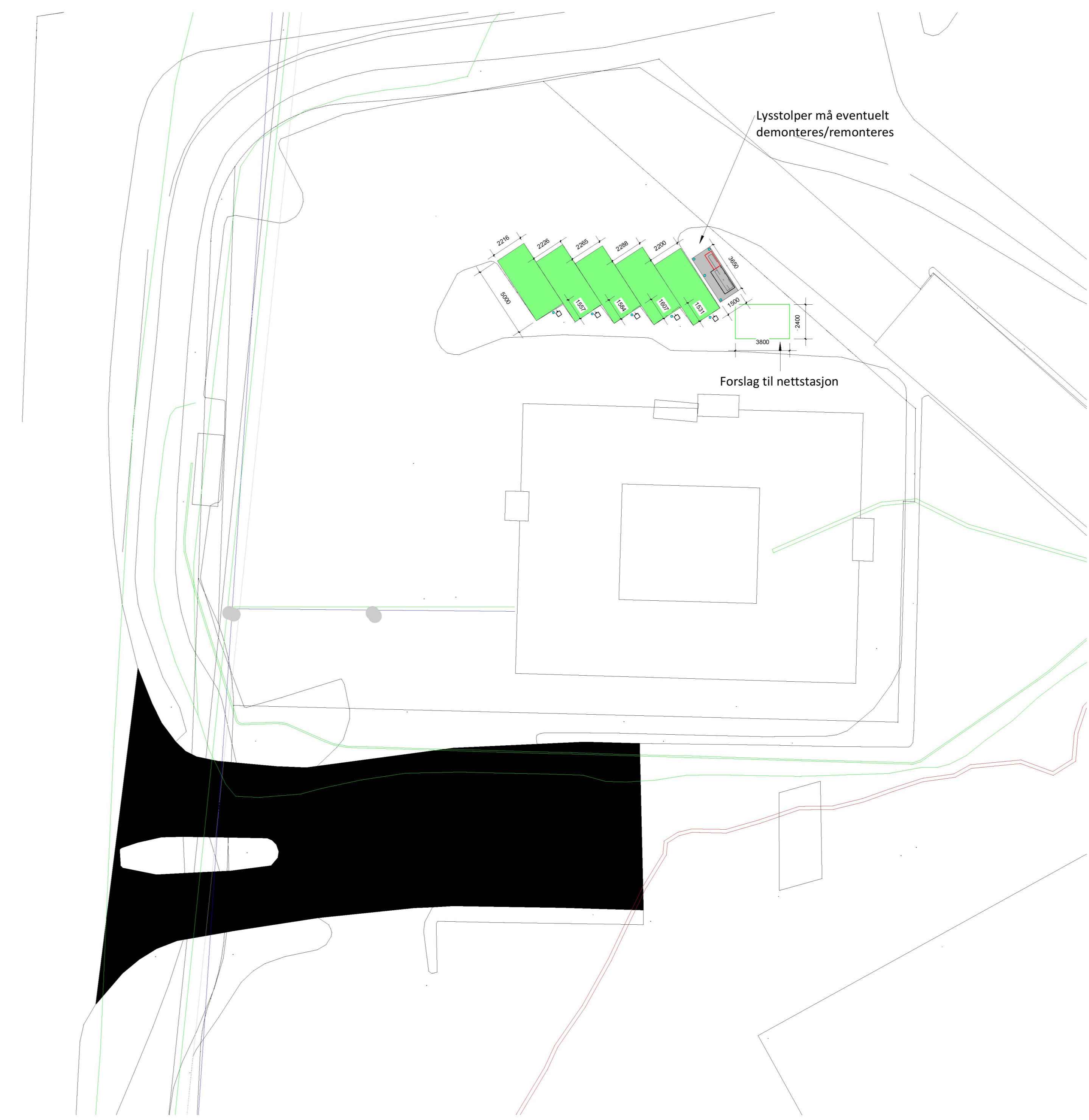
Elektro Oversiktsplan - 279 McDonalds Karmøy 1_200
