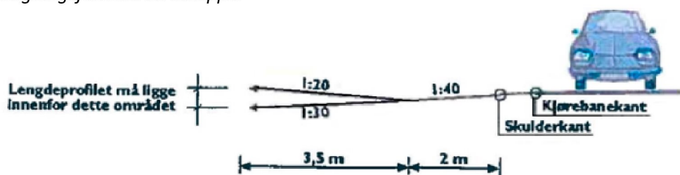
Figur 2: Lengdeprofil
