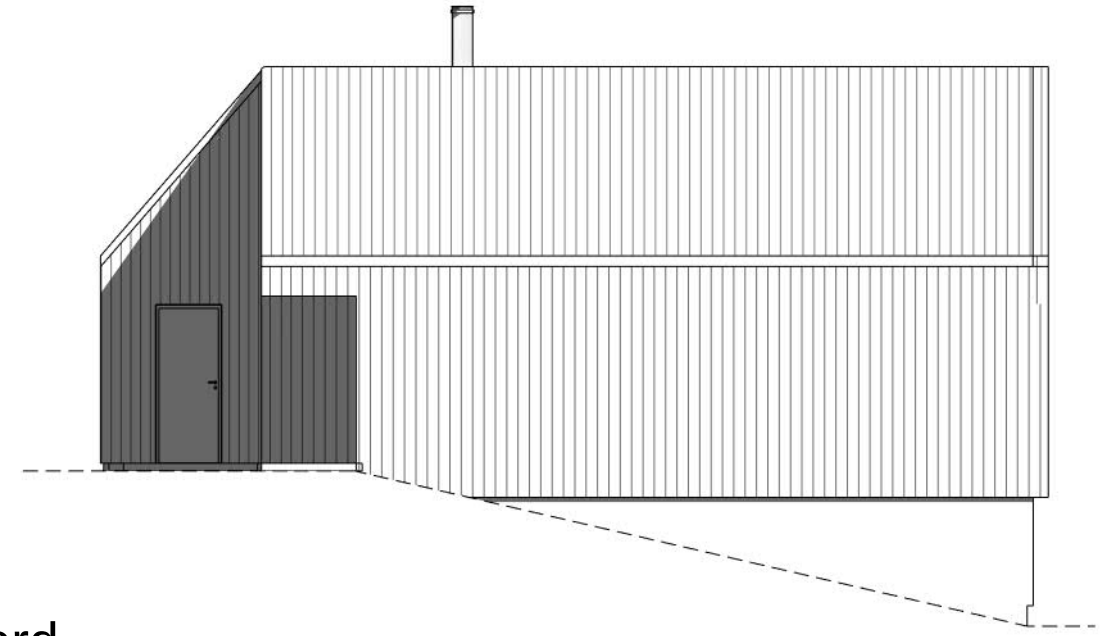
Nord 1 : 100
