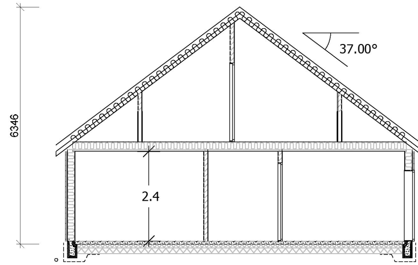
Snitt A:A
