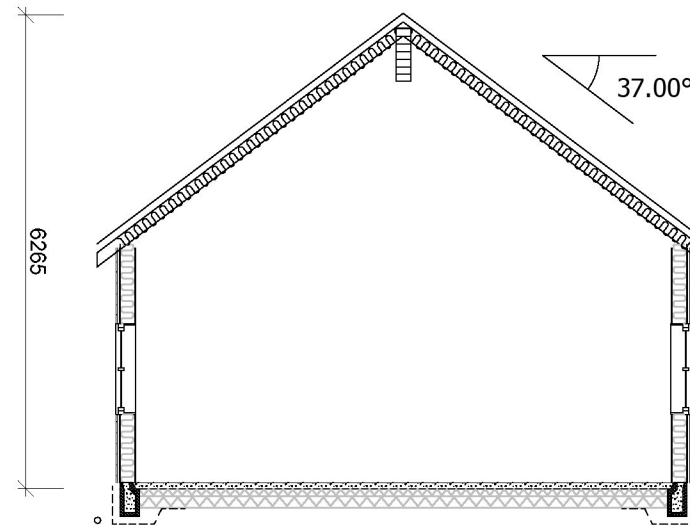
Snitt B:B
