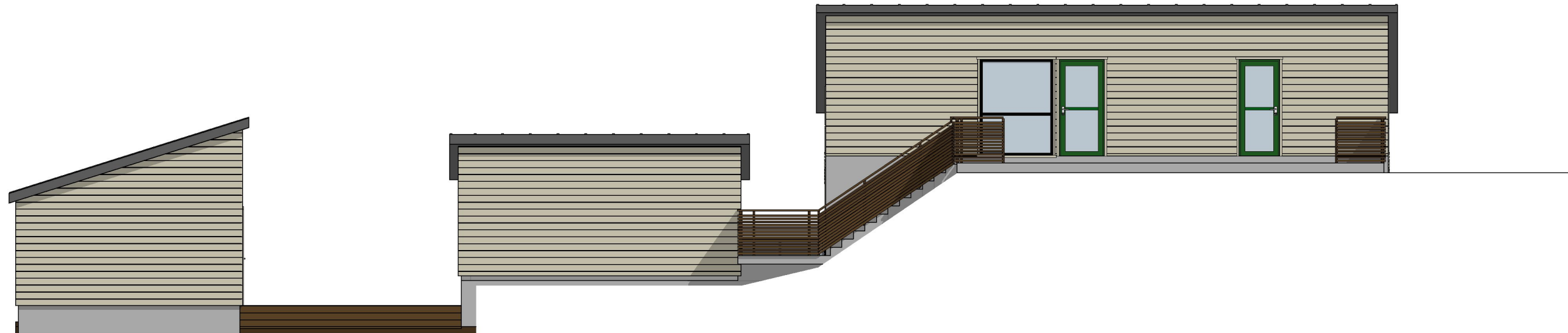
1:100 Fasade Øst
