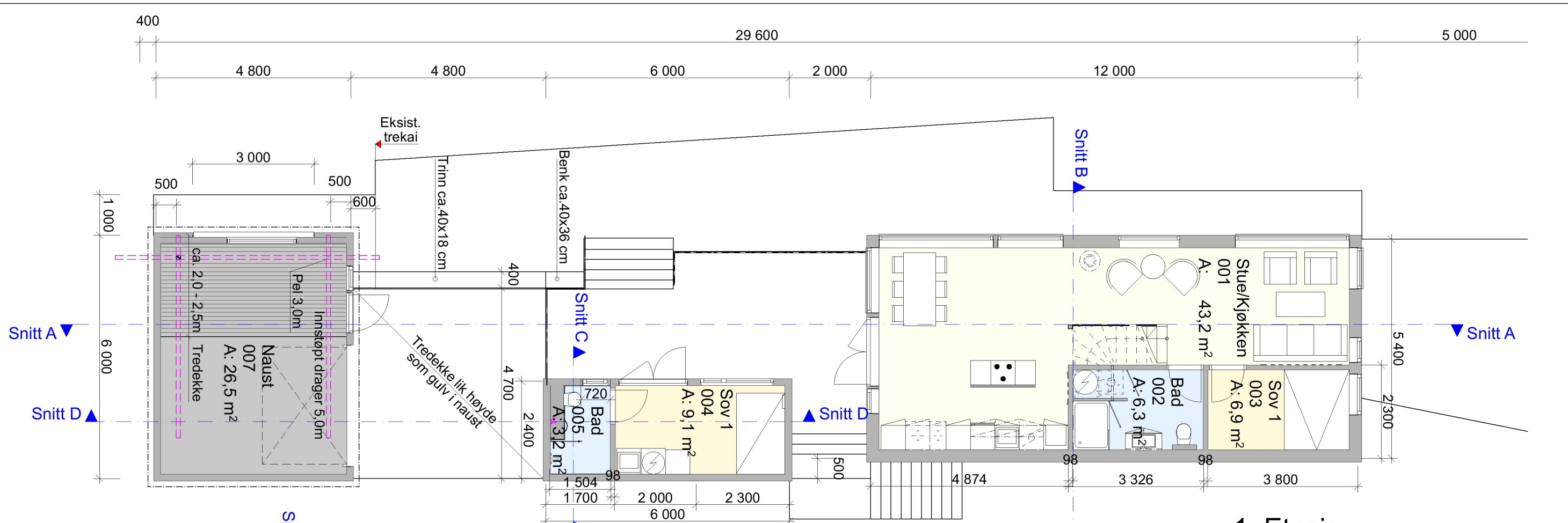
1. Etasje
