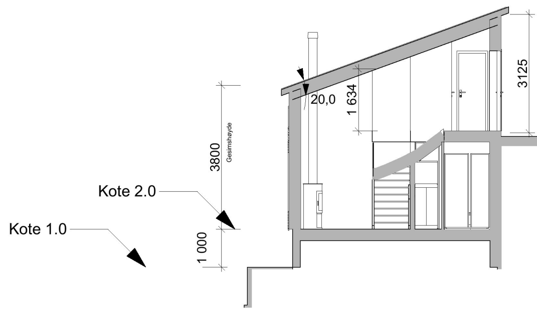
1:100 Snitt B
