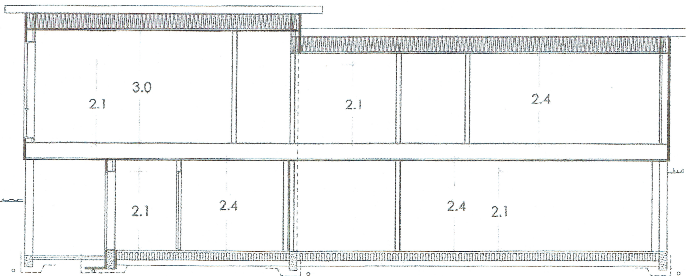
Snitt A-A
