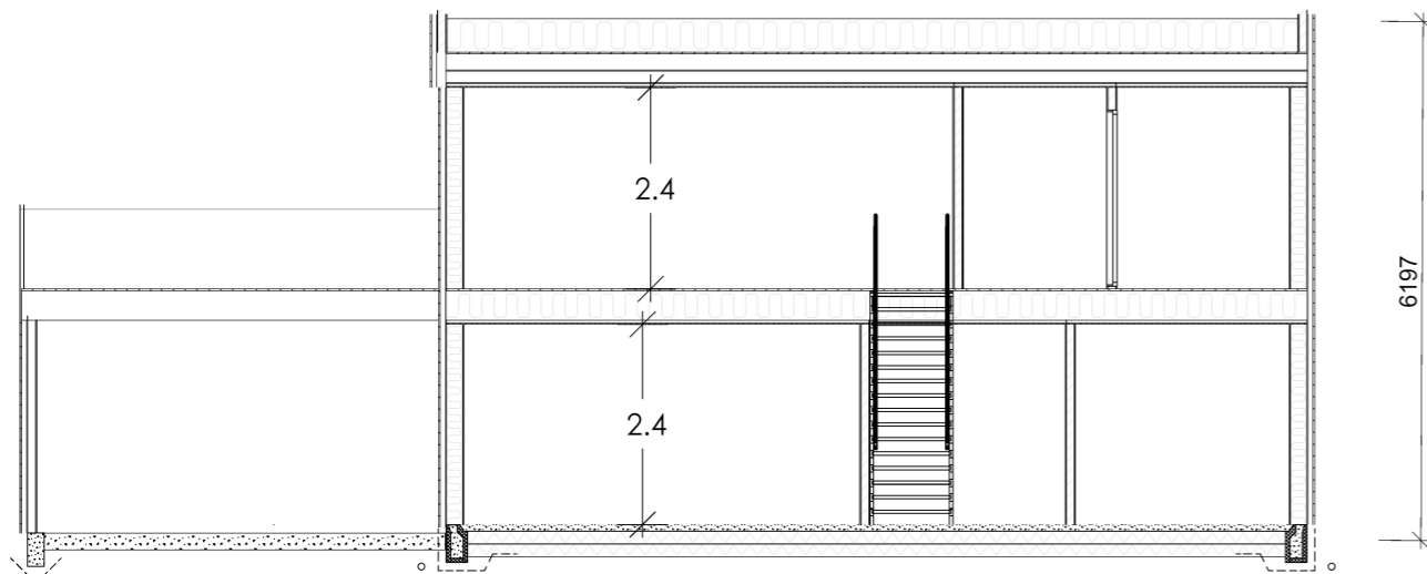
Snitt A:A
