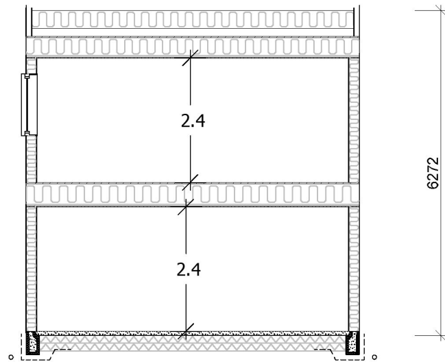
Snitt B:B
