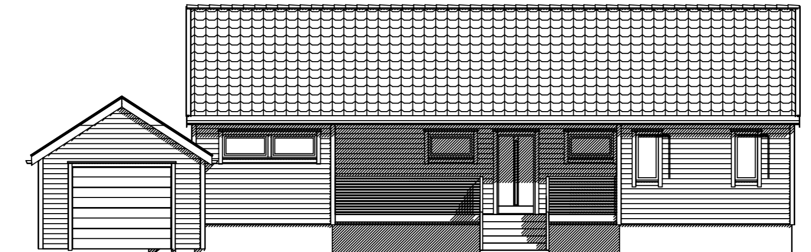
Fasade øst
