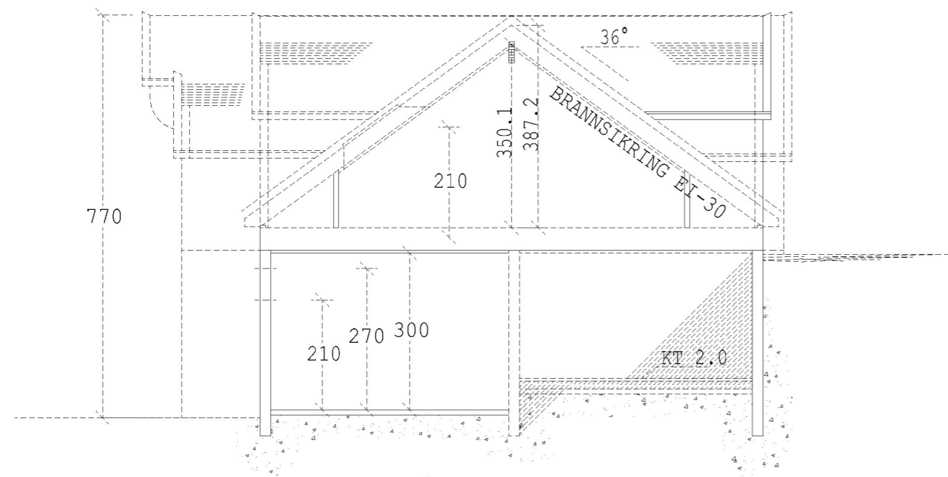
SNITT A-A
