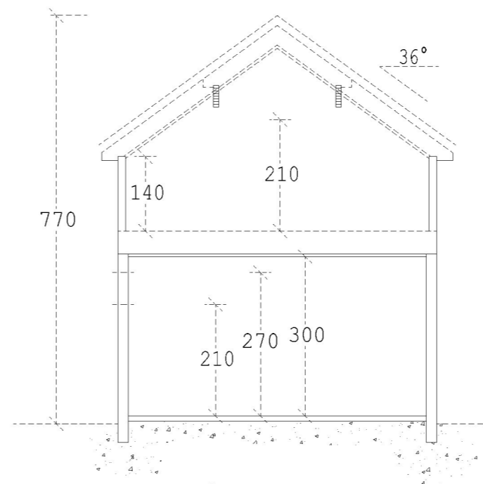
SNITT B-B
