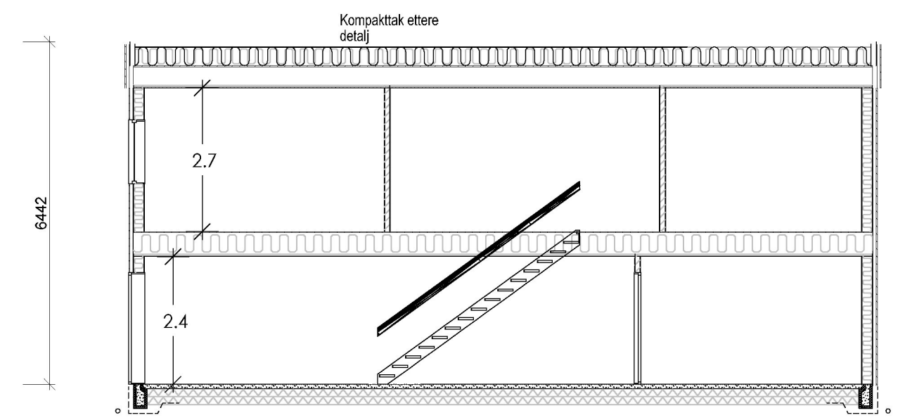
Snitt A:A
