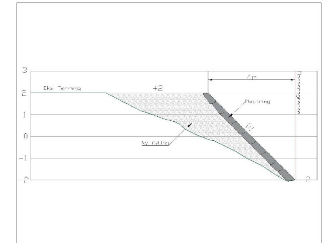
Teknisk prinsipp snitt - målestokk 1:10
