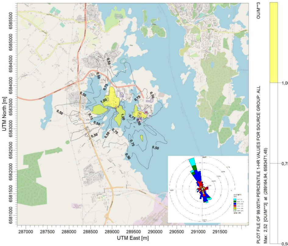
Figur 2: Luktspredningskart for juni måned. Områder som er gule har luktkonsentrasjon over 1 \text{ ouE/m}^3 . Ingen boliger ligger i gult område. Vindrosen for juni er vist i nedre høyre hjørne.
