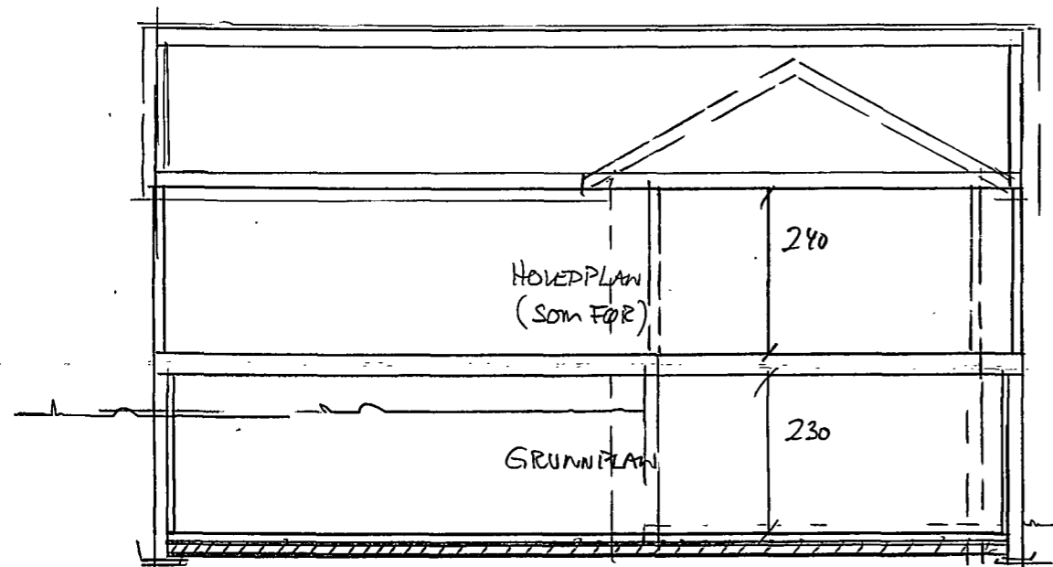
SNITT
