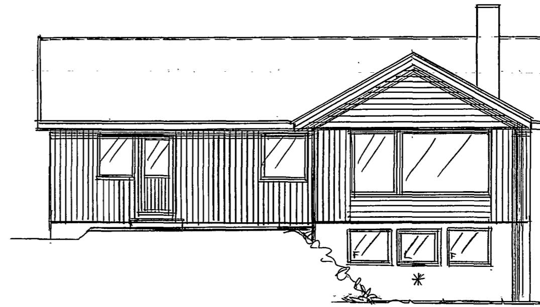
FASADE SØR
