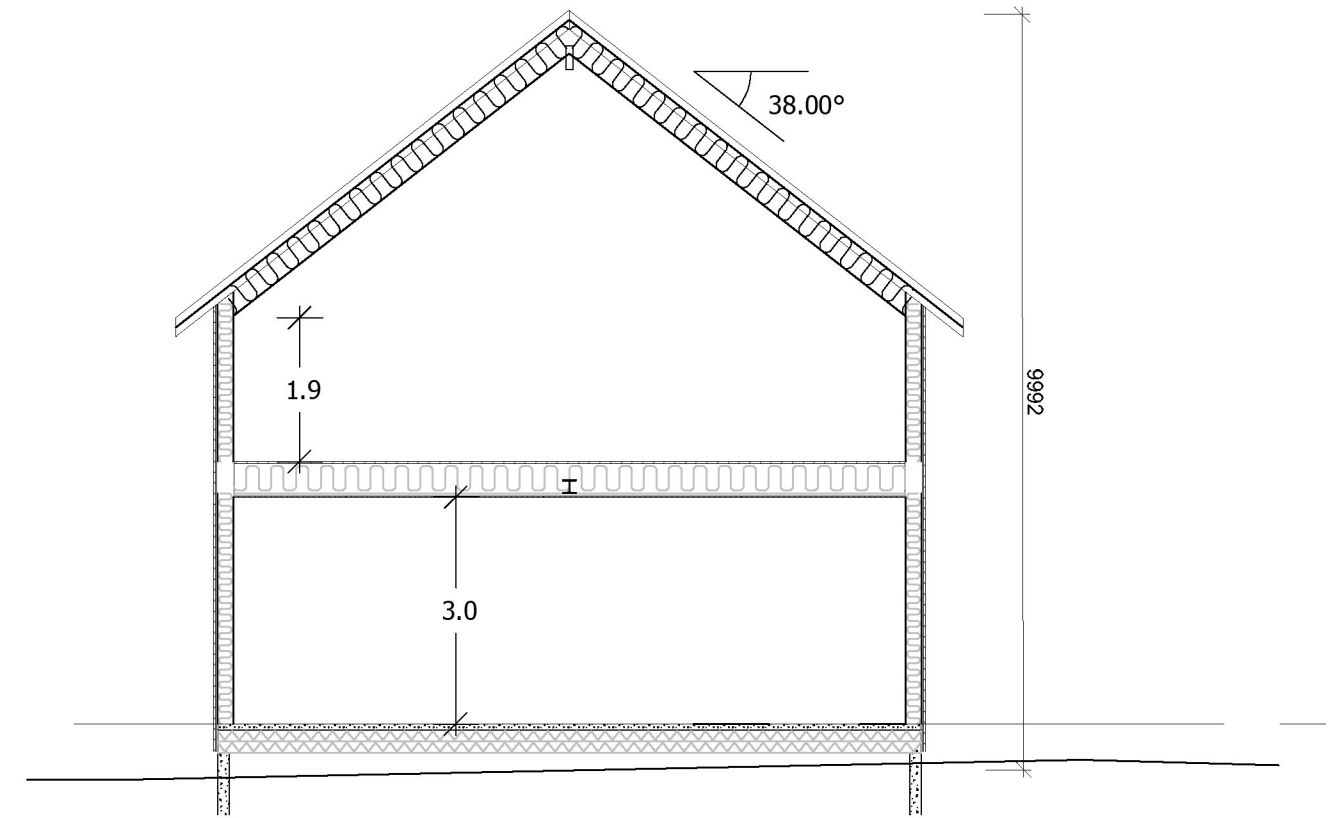
Snitt A:A
