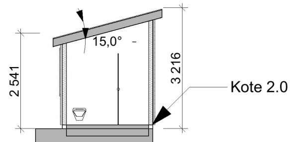
Snitt C
