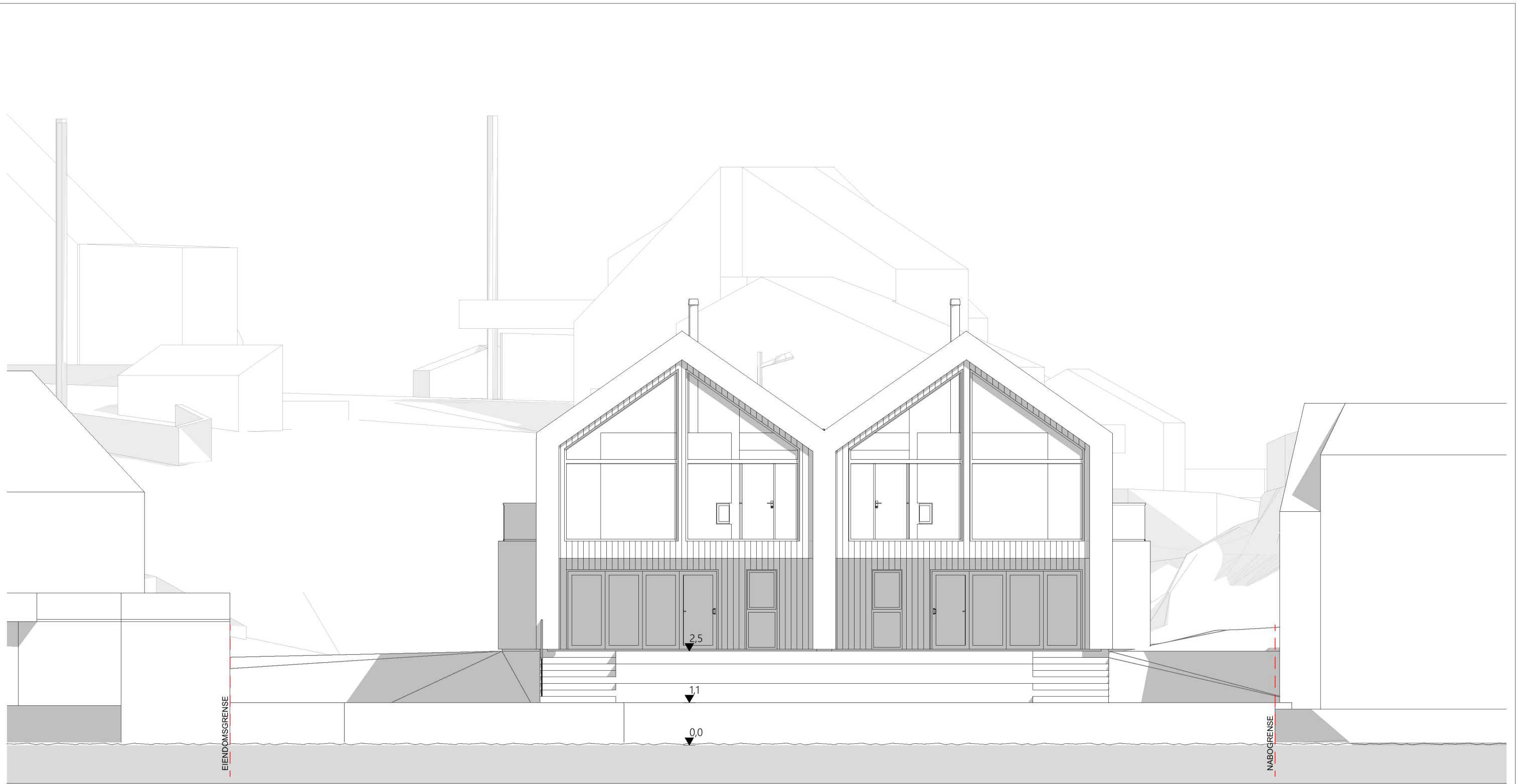
FASADE VEST
