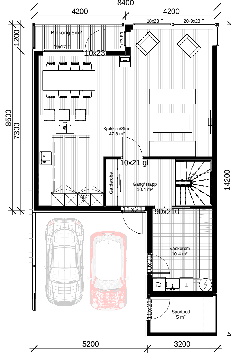
Et. 2 1 : 100
