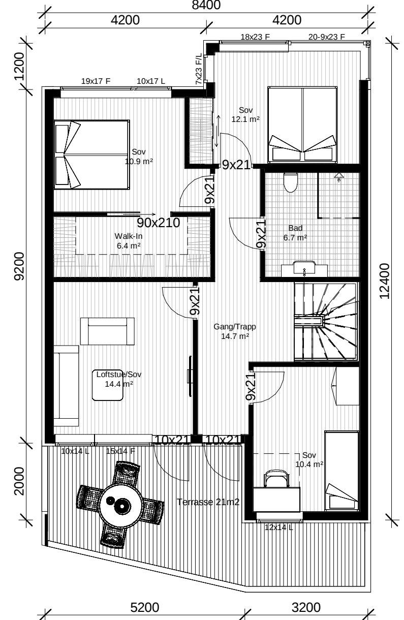
Et. 3 1 : 100
