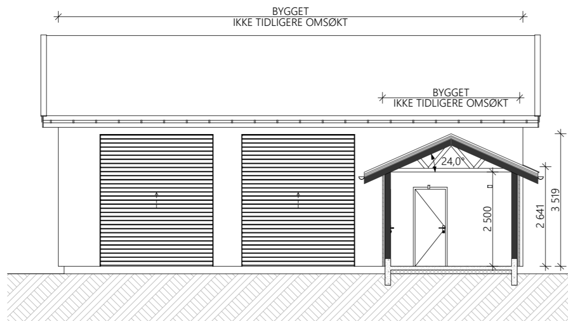
SNITT B-B
