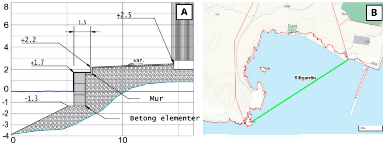
Figur 1: Illustrasjon av utforming av bryggefront (A) og plassering av siltgardin over Visnesbukta (B). Kilde: søknad om endring av tillatelse.
