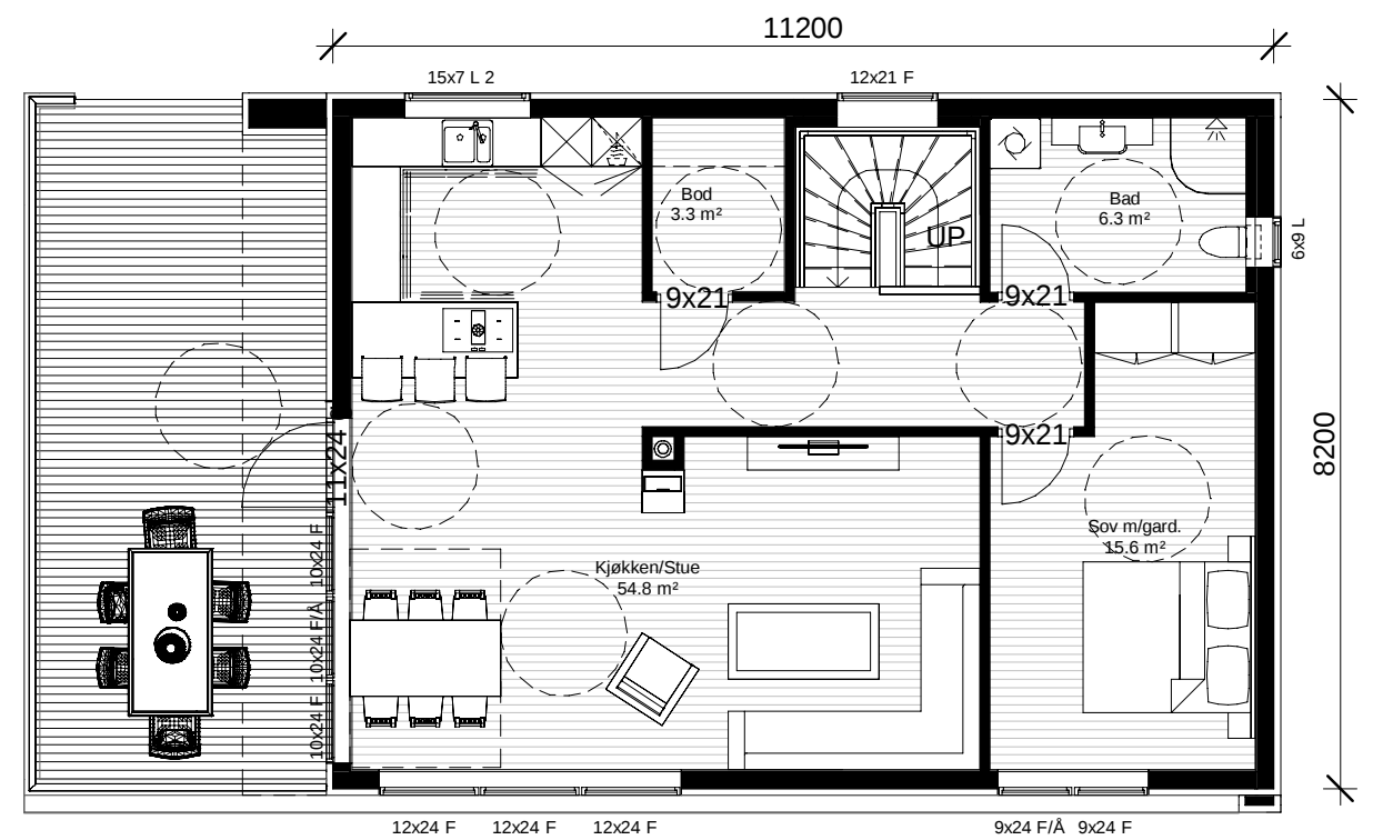
Et. 2 1 : 100
