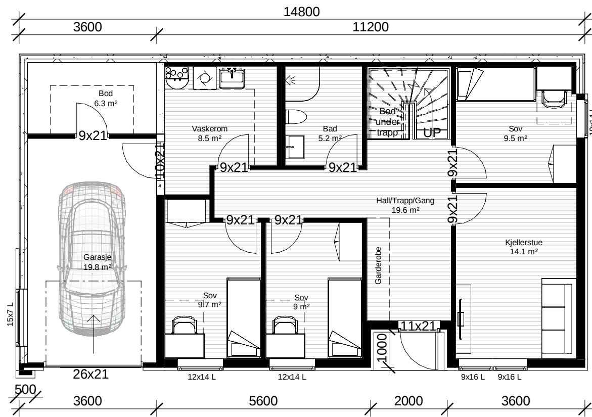
Et. 1 1 : 100
