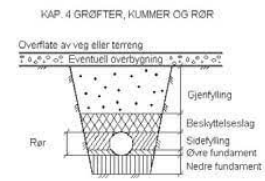
Prinsippskisse profil grøft
